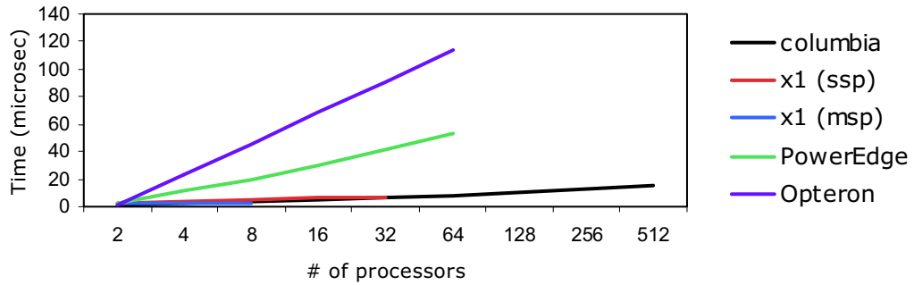
Fig. 4. MPI_Barrier
